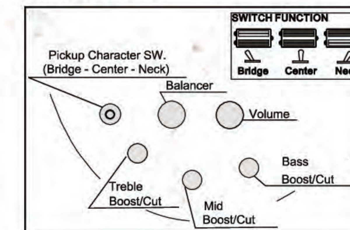
ATK N3 3-band EQ
