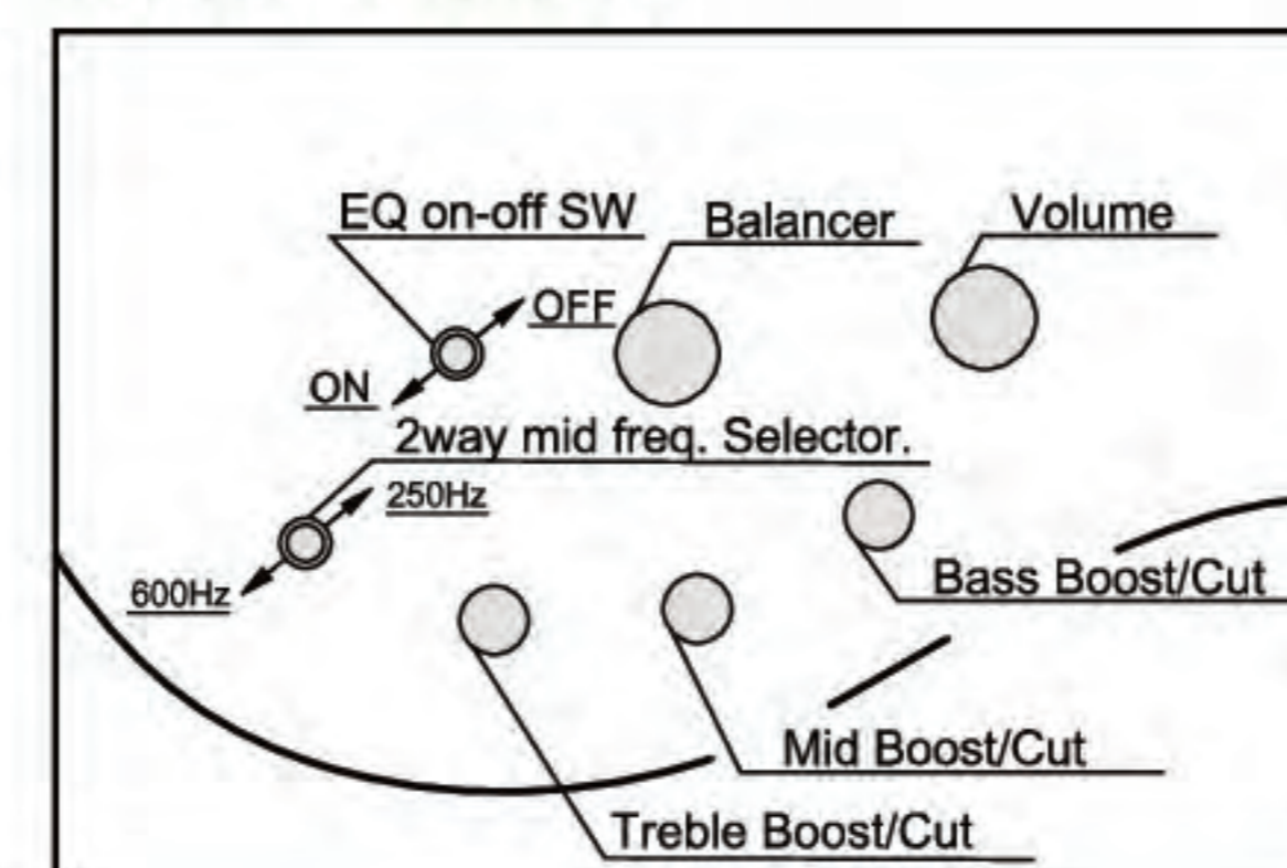
EQB-IIISC 3-band EQ
