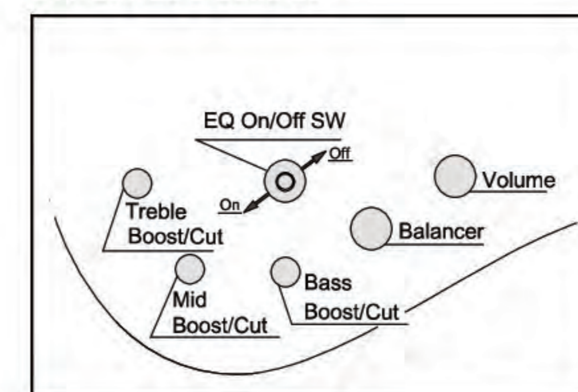
E4 / E5 / E6 3-band EQ
